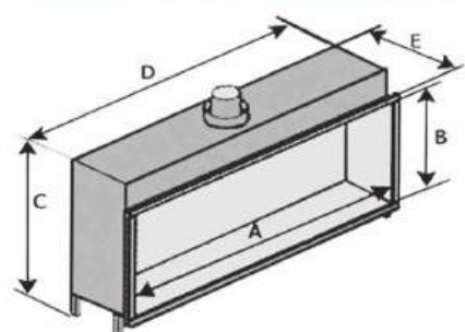
Salida de humos central
